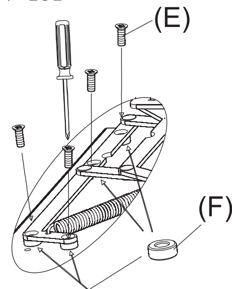
힌지 조립방법
